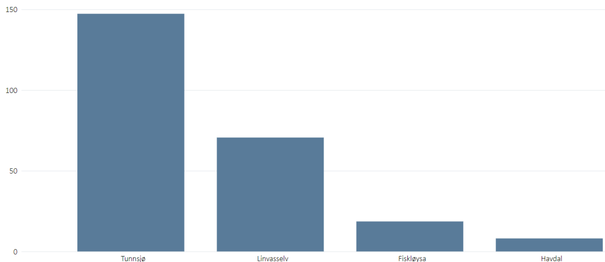
Figur 4.3.2 Årlig middelproduksjon GWh per vannkraftverk i Lierne. Tunnsjø 147,3, Linvasselv 70,6, Fiskløysa 18,6 og Havdal 8,1 GWh.
